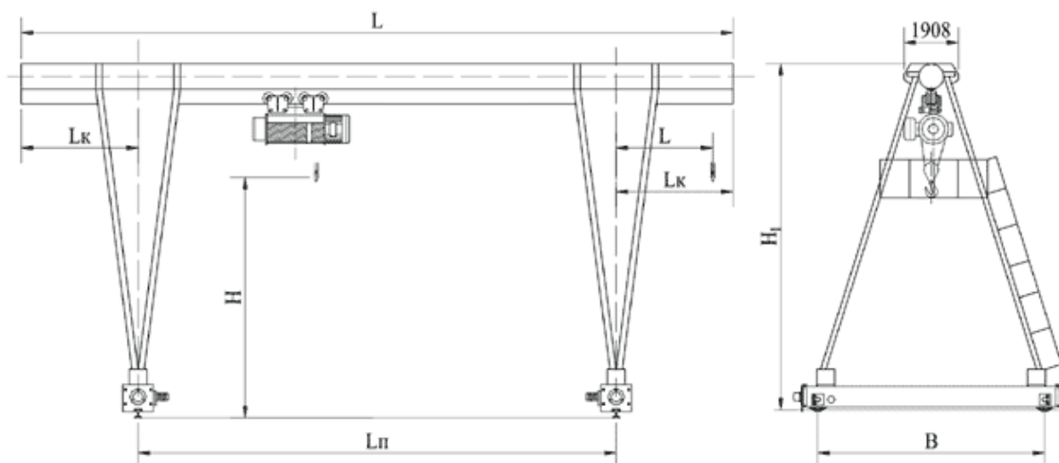
Рис. 1 Общий вид крана Технические характеристики
