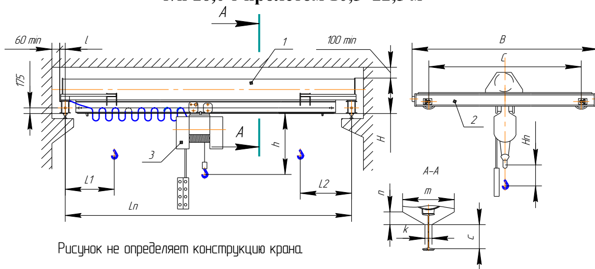
Рис. 1 Общий вид крана:
