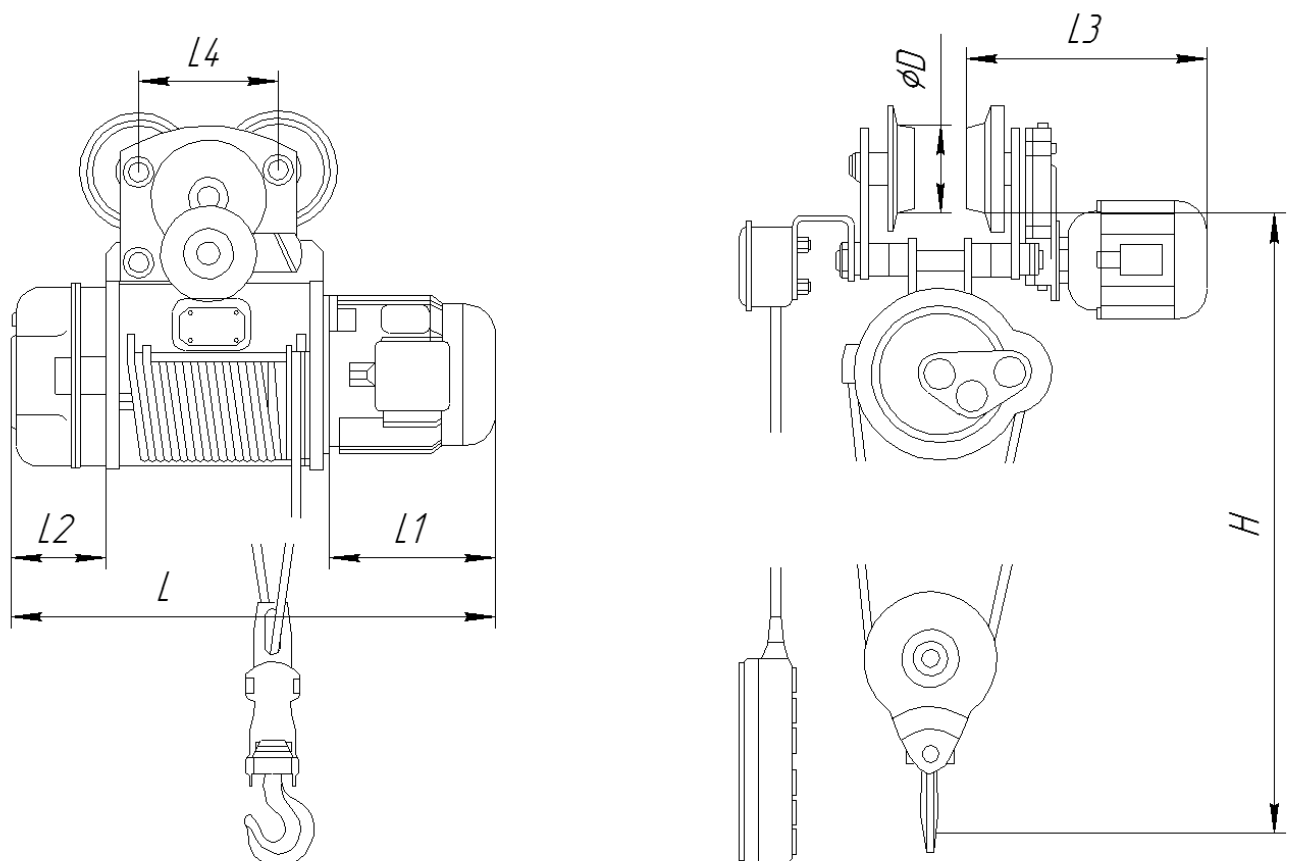
Рис. 1. Таль электрическая канатная передвижная грузоподъемностью 1 т, высотой подъема 6,0÷30,0 м
